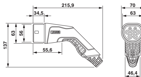
Maßzeichnung Fahrzeug-Ladestecker
