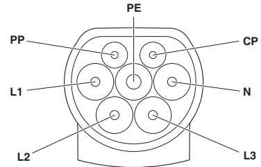
Pinbelegung Infrastruktur-Ladestecker
