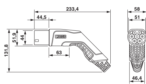
Maßzeichnung
